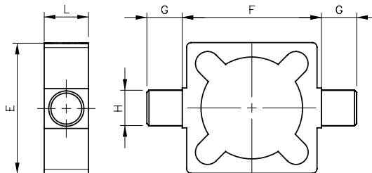
Výkyvné upevnenie
