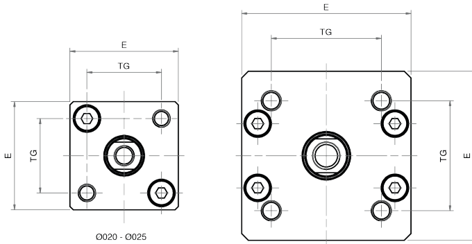
Ø032 - Ø040 - Ø050 - Ø063 - Ø080
