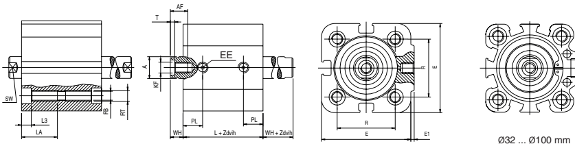
Ø12 ... Ø25 mm
